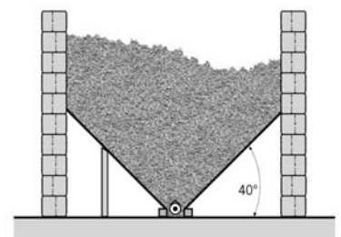
Rutschschräge 40° im Pelletslager mit glatter Oberfläche
